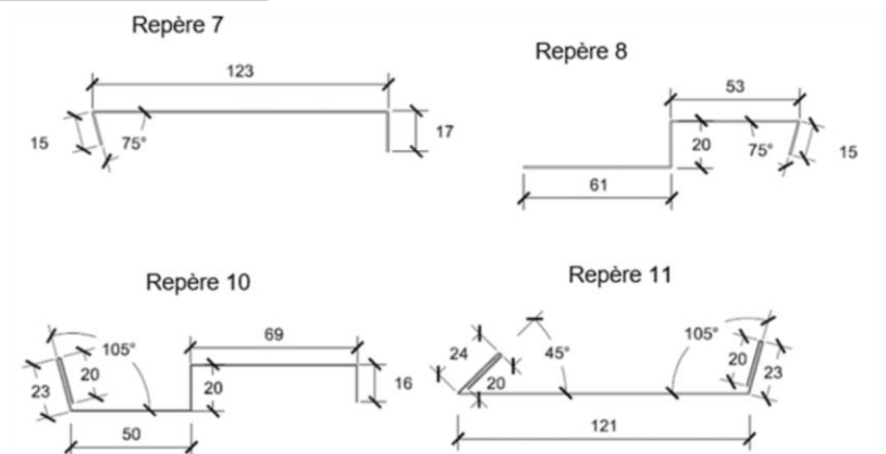
Figure 16 – Joint de dilatation - pose horizontale et pose verticale (déplacement maxi de 20 mm)
