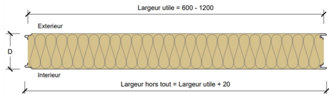
Figure 1 bis - Emboîtement
