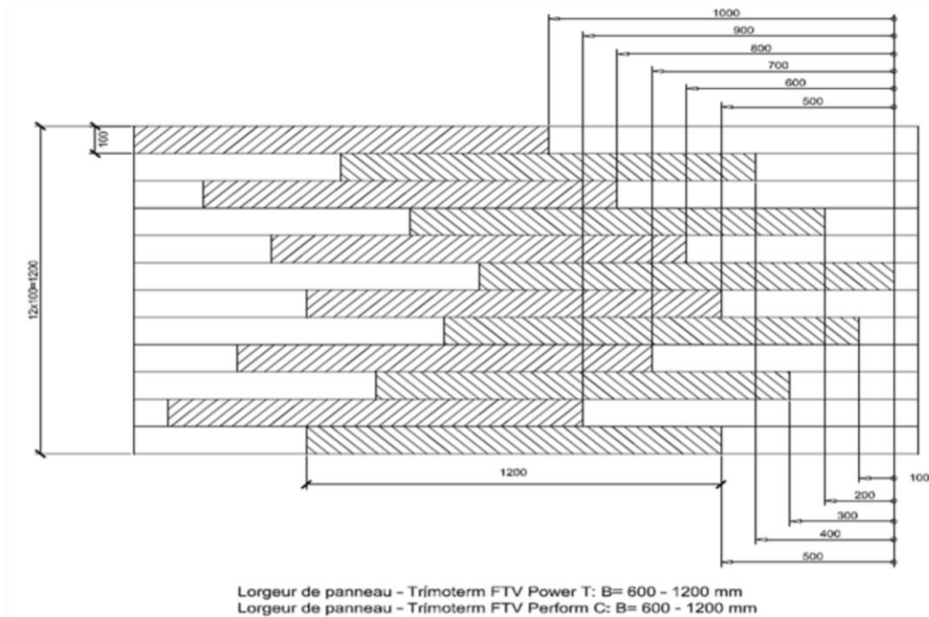
Figure 1 – Géométrie des parements et mise en place des lamellas
