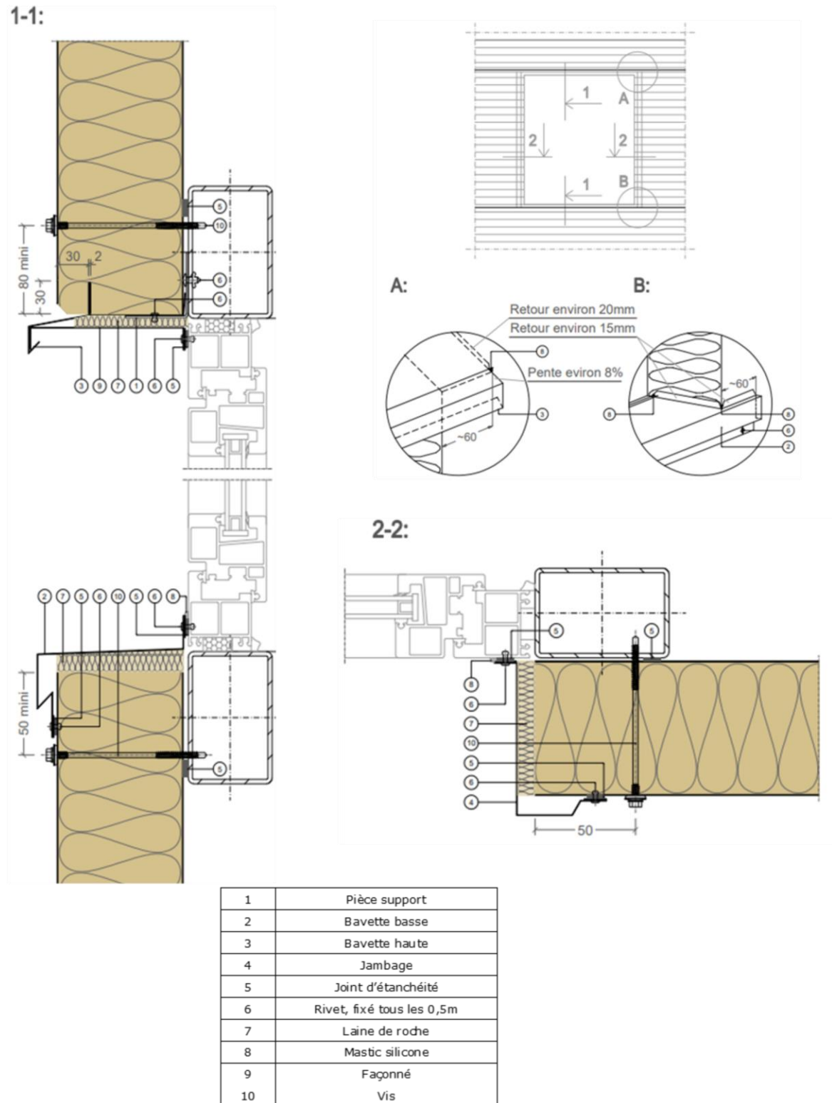
Figure 15 - Baie en pose verticale
