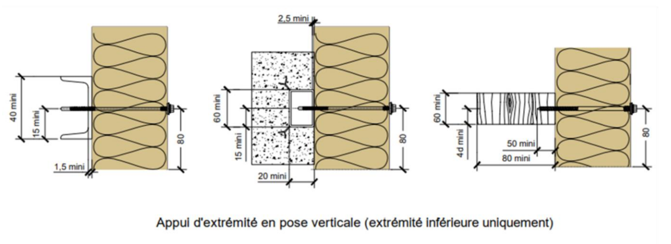
Figure 2 – Dimensions minimales des appuis
