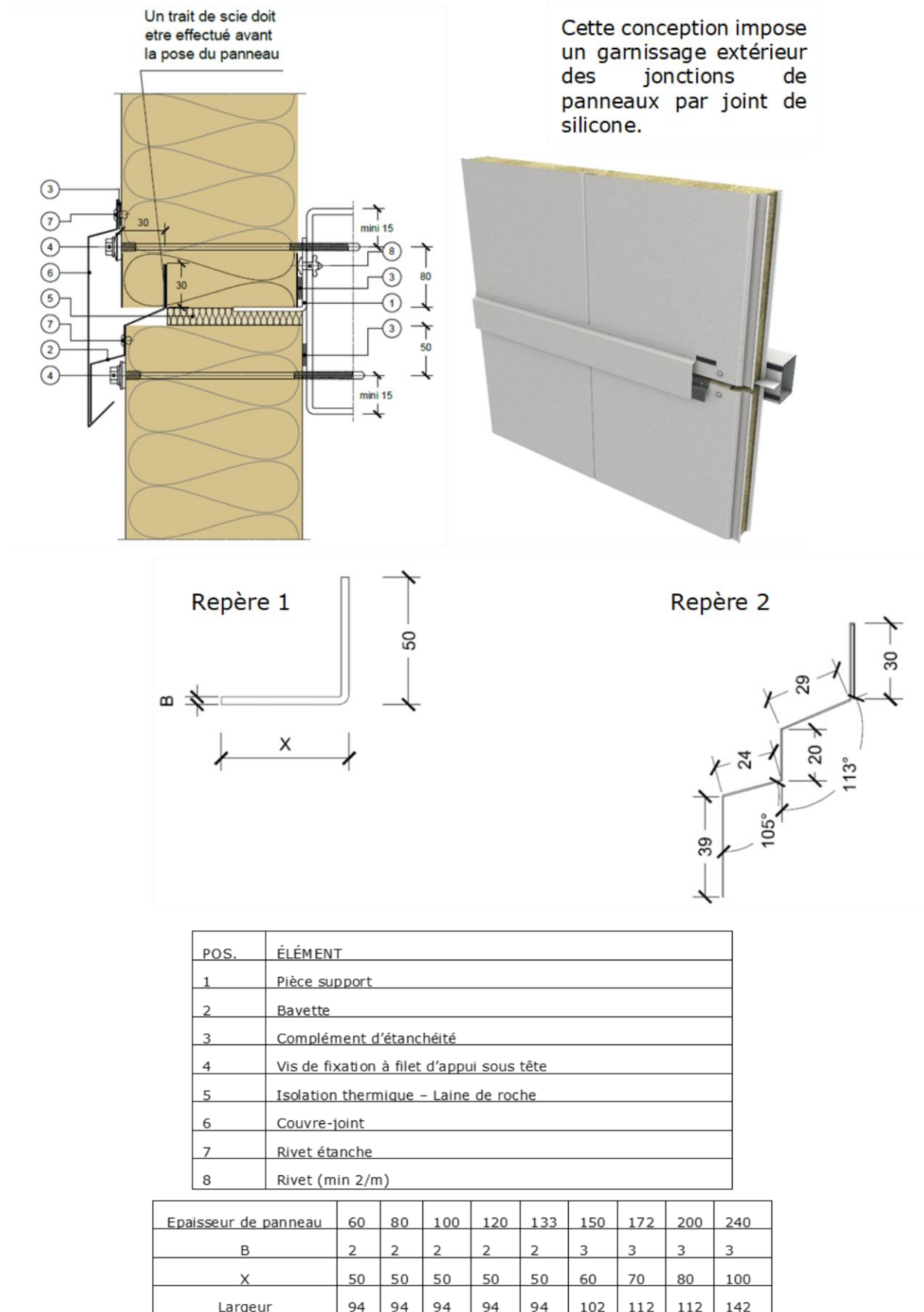
Figure 4 - jonction horizontale en pose verticale
